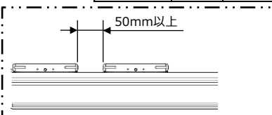
図6：追加テーブルの最小距離 テーブル間は50mm以上離してください。 有効ストロークは追加テーブル全長とテーブル間を離れた距離が減少します。
