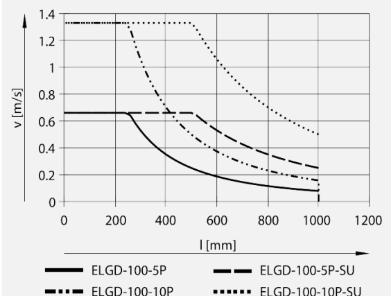
図5：ストローク-許容速度特性
