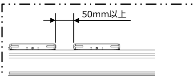
図6：追加テーブルの最小距離
