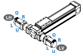
図1：モータ取付位置とケーブルの向き
