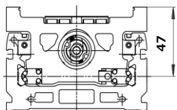
図3：ガイド中心からテーブル取付面までの高さ 許容モーメントや強度限界を検討する際は、この高さを考慮して計算ください。
