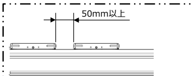
図4: 追加テーブルの最小距離
