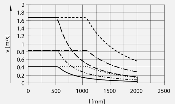
図5：ストローク・許容速度特性（標準テーブル）
